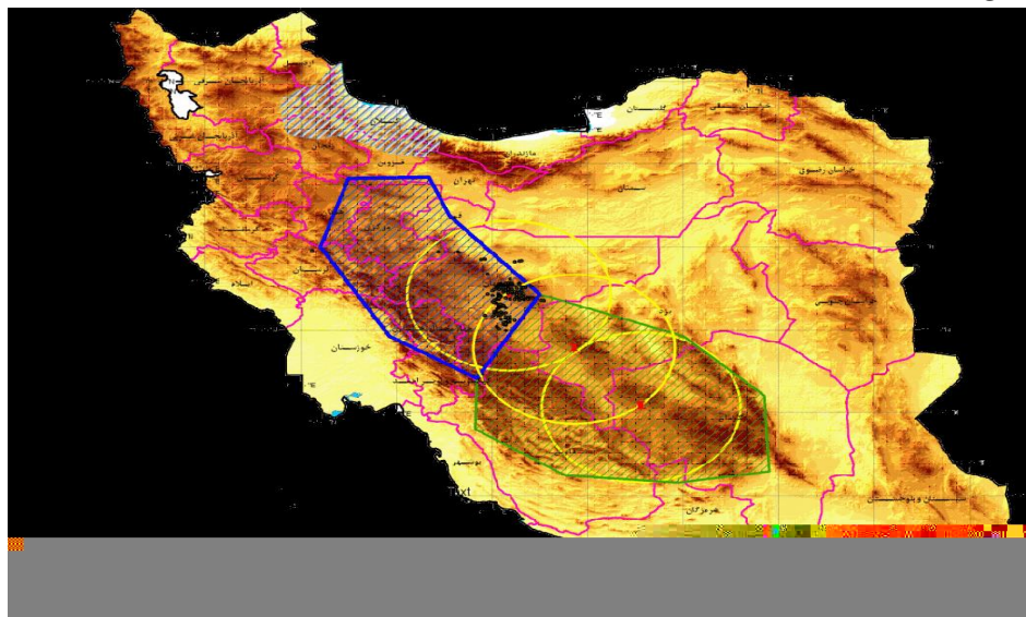
شکل ۶: محدوده سبزرنگ پروژه "فلات مرکزی"، محدوده آبی رنگ پروژه "زاگرس" و محدوده سفیدرنگ پروژه گیلان می باشد.
